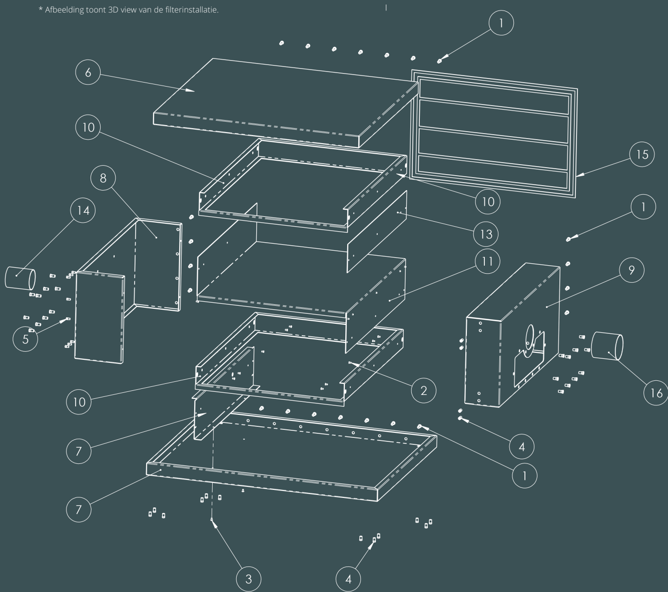
* Afbeelding toont 3D view van de filterinstallatie.
